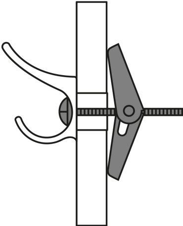
Fijación en paredes huecas o delgadas
